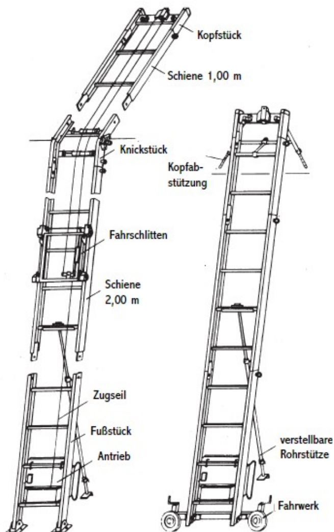
Šikmý výtah s ohybem a střešními nástavci postavený na patkách
